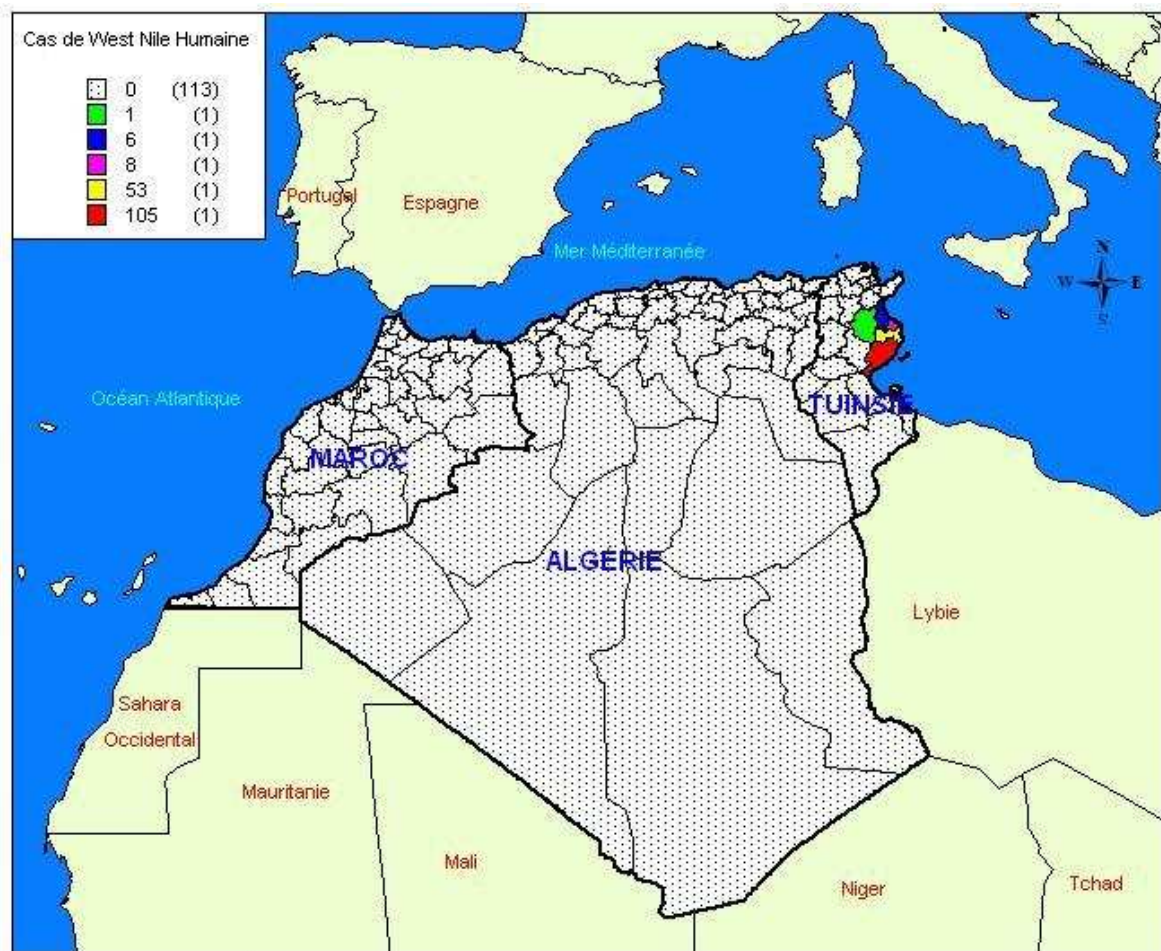
ZONES DE DETECTION DE LA WEST NILE HUMAINE AU MAGHREB EN 1997
